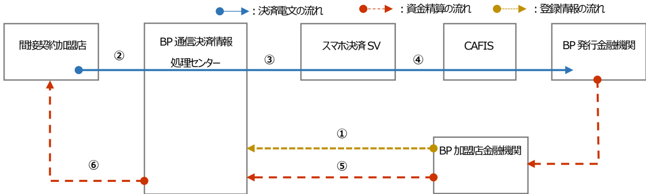
図2:BP 通信情報処理センターにおける情報登録・設定・資金精算フロー
