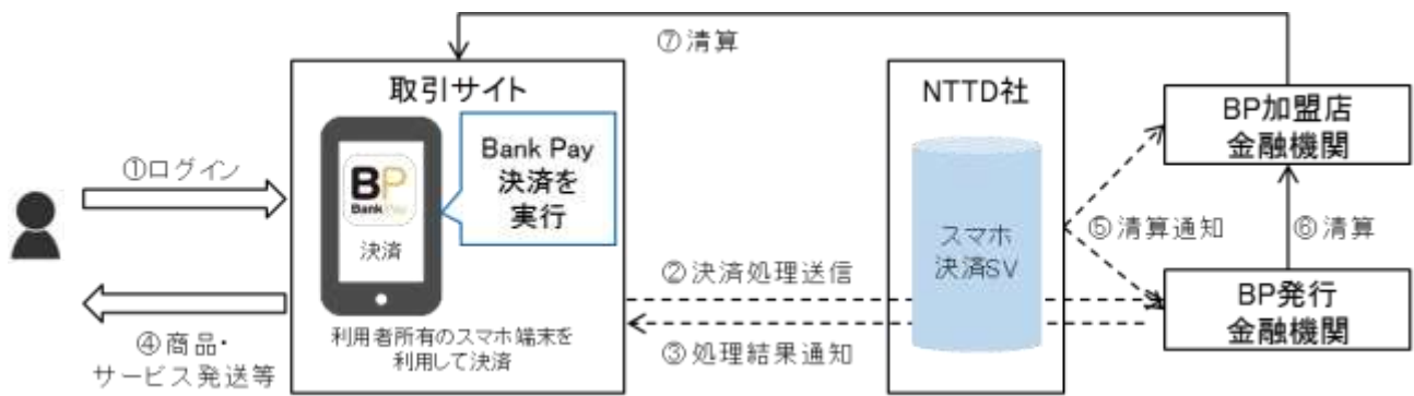
図5:直接決済方式で取引を行う場合(BP 提携利用者アプリ利用時)
