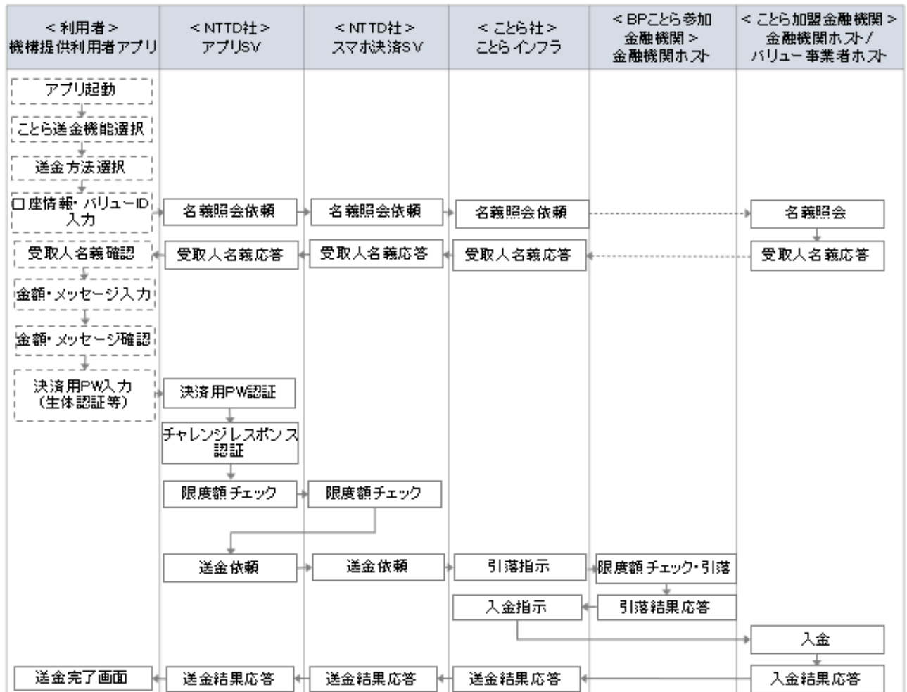
図 2 : 口座番号指定送金・バリュー ( Pay 事業者 ) 指定方式の送金取引の流れ
