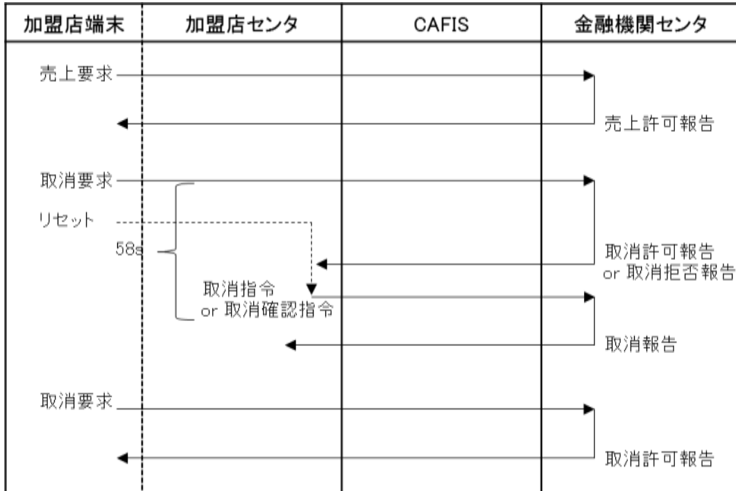
図1:事例 タイムアウト前にBP 加盟店等側がリセットを行ってしまった場合の処理について
